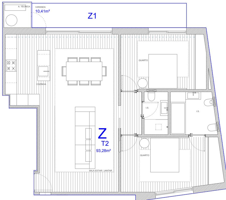
HABITAÇÃO PLANTA PARCIAL DO PISO 2 Escala: 1:100
