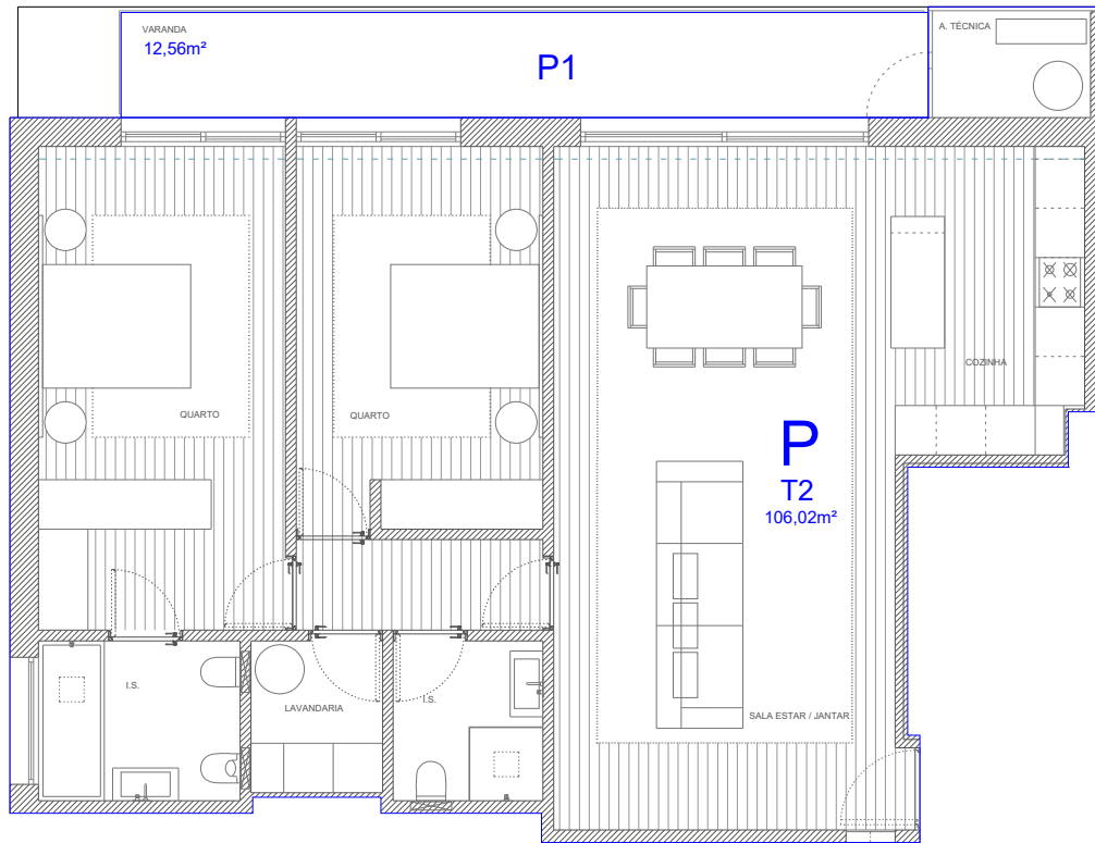
HABITAÇÃO PLANTA PARCIAL DO PISO 1 Escala: 1:100
